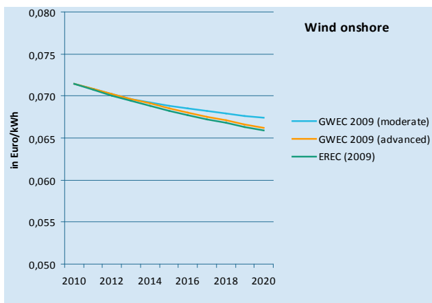
Abbildung 18: Sensitivitätsanalyse für Wind onshore mit 2000 Voll- laststunden.
