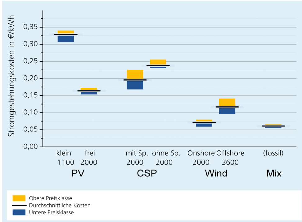
Abbildung 4: Vergleich der Stromgestehungskosten (2010) für PV, CSP und WEA. Der Wert unter der Technologie bezieht sich bei den Solartechnologien auf die jährliche Einstrahlung am Kraftwerksstandort, bei Windkraft auf die jährliche Volllaststundenanzahl.
