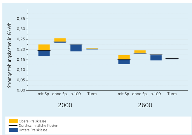
Abbildung 9: Stromgestehungskosten für CSP nach Anlagentyp und Einstrahlung (2010).
