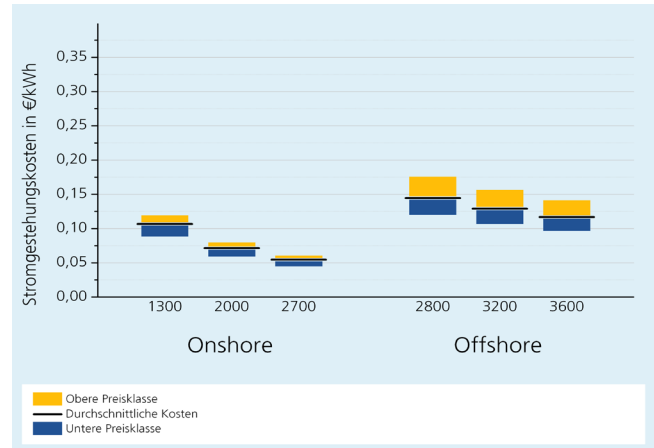
Abbildung 12: Stromgestehungskosten für WEA nach Standort und Volllaststunden (2010).
