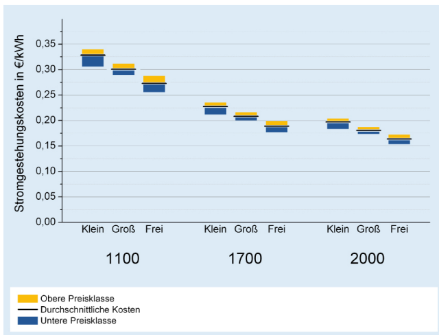
Abbildung 6: Stromgestehungskosten für PV nach Anlagentyp und Einstrahlung (2010).
