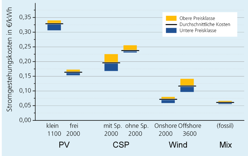
Abbildung 1: Vergleich der Stromgestehungskosten (2010) für PV, CSP und WEA. Der Wert unter der Technologie bezieht sich bei den Solartechnologien auf die jährliche Einstrahlung am Kraftwerksstandort, bei Windkraft auf die jährliche Volllaststundenanzahl.
