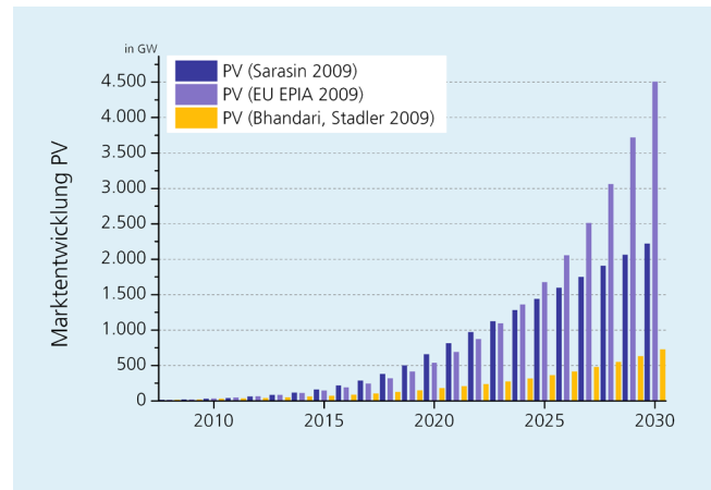
Abbildung 5: Marktprognose der kum. Kraftwerksleistung für PV 2010-2030 nach Sarasin 2009, EPIA 2010, Bhandari/Stadler 2009.
