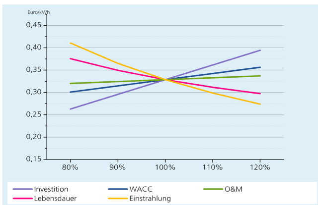
Abbildung 7: Sensitivitätsanalyse PV-Kleinanlage mit Energieertrag 900 kWh/kWp (2010), 100% entspricht Mittelwert für PVklein aus Abb.4.
