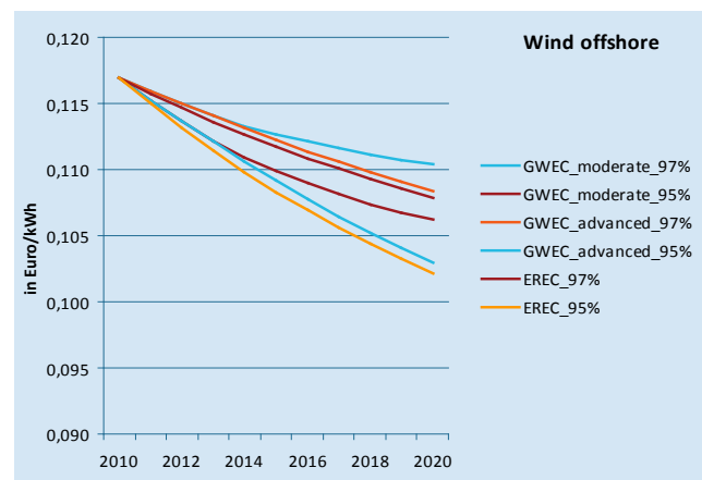
Abbildung 19: Sensitivitätsanalyse für Wind offshore mit 3600 Voll- laststunden.
