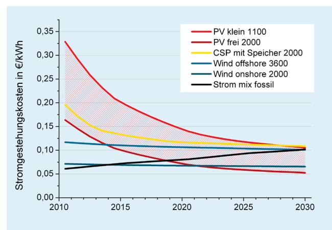
Abbildung 14: Prognose für Stromgestehungskosten für EE anhand Lernkurven bis 2030.
