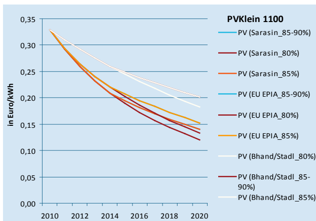
Abbildung 16: Sensitivitätsanalyse für PVklein mit 1100 kWh/kWp.
