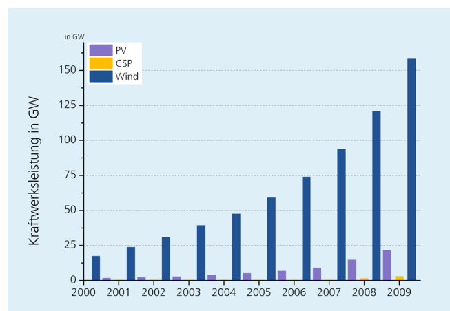
Abbildung 3: Globale installierte Kapazität 2000-2009 nach GWEC 2009, Sarasin 2009.
