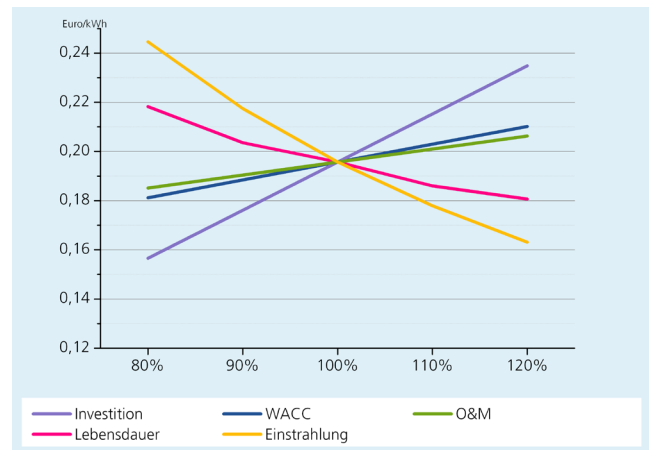
Abbildung 10: Sensitivitätsanalyse CSP (50MW mit Speicher) mit jährlicher Einstrahlung von 2000 kWh/m 2 /Jahr (2010), 100% entspricht Mittelwert für PVklein aus Abb.4.
