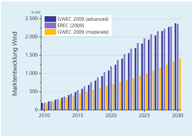
Abbildung 11: Marktprognosen kumulierter Windkraft 2010-2030 nach GWEK 2009, EREC 2009).
