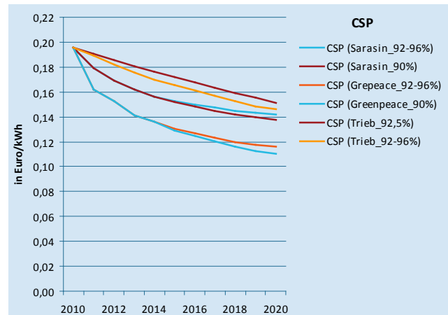
Abbildung 15: Sensitivitätsanalyse für CSP mit Speicher und 2000 kWh/m 2 /Jahr.
