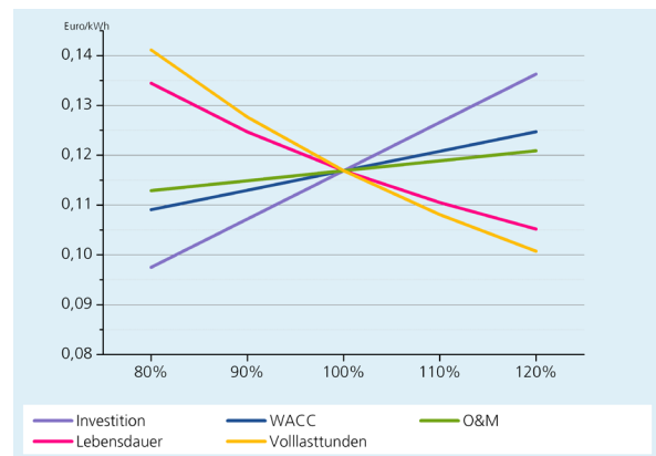
Abbildung 13: Sensitivitätsanalyse Wind-Offshore-Anlage mit 3600 Volllaststundenzahl, spezifische Investition von 3200 Euro/kW.
