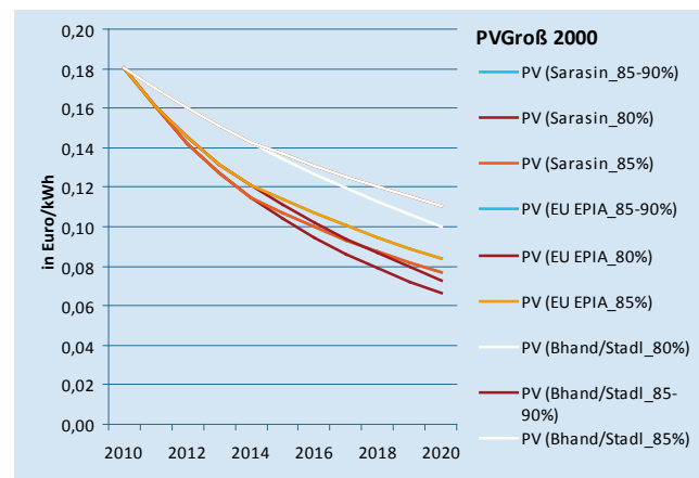
Abbildung 17: Sensitivitätsanalyse für PVGroß mit 2000 kWh/kWp.
