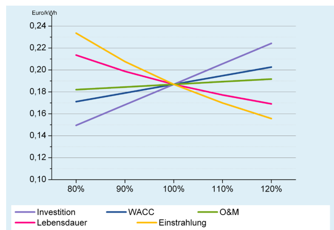
Abbildung 21: Sensitivitätsanalyse für CPV
