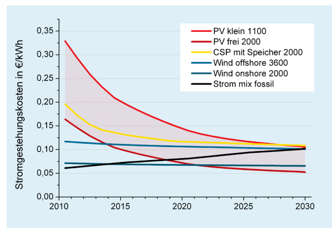
Abbildung 2: Lernkurvenbasierte Prognose von Stromgestehungskosten erneuerbarer Energien bis 2030.
