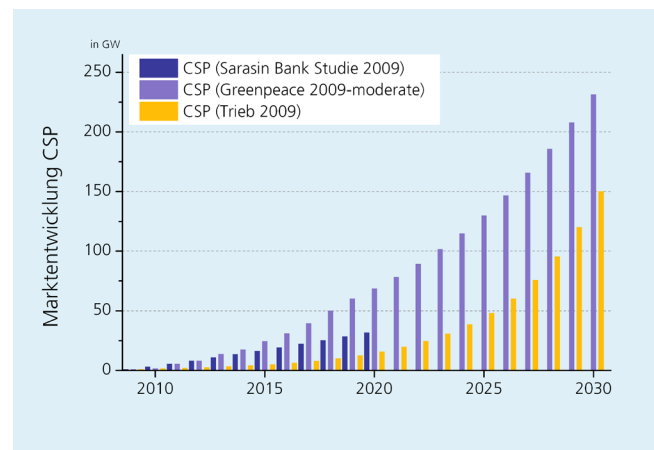
Abbildung 8: Marktprognose der kumulierten Kraftwerksleistung für solarthermische Kraftwerke 2010-2030, Sarasin (2009), Trieb (2009), Greenpeace (2009).
